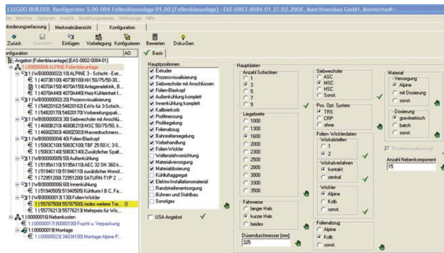
Konfigurator für Folienblasanlagen mit Erfassung der Basisanforderungen
